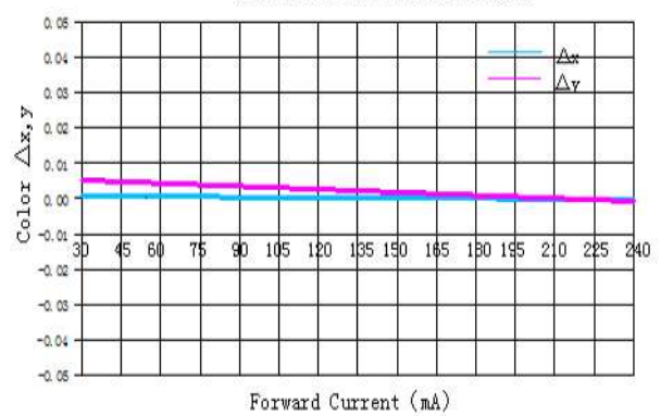
Forward Current vs. Color \Delta x, y 电流与色坐标偏移量曲线关系
