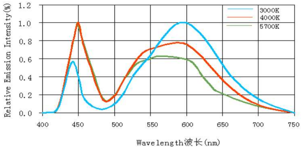
Spectrum Distribution 光谱分布图
