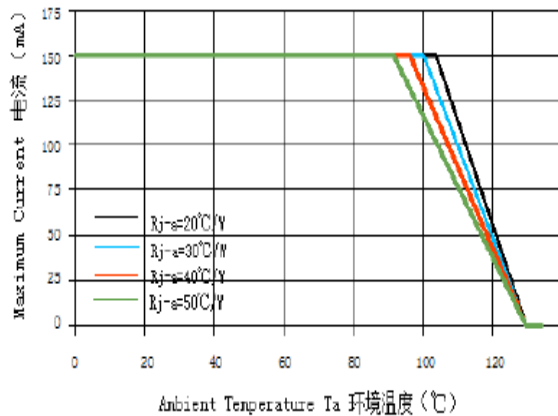
Thermal design 电流与环境温度曲线关系
